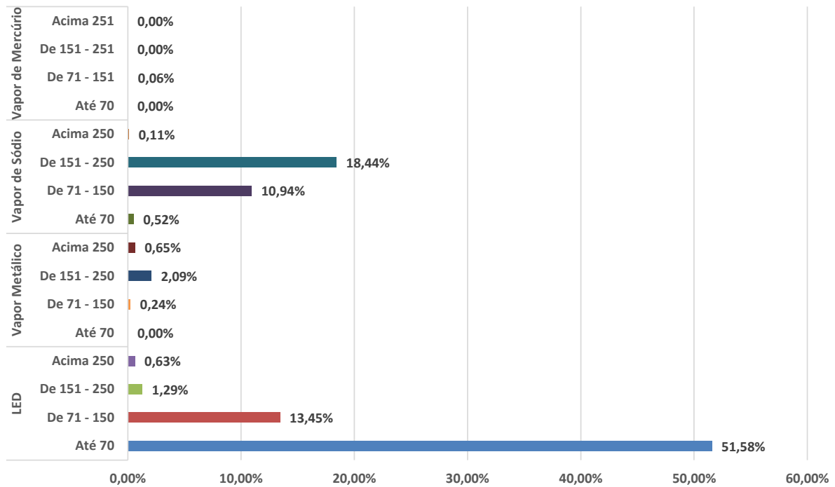
% Distribuição Tecnologia por Faixa de Potência
